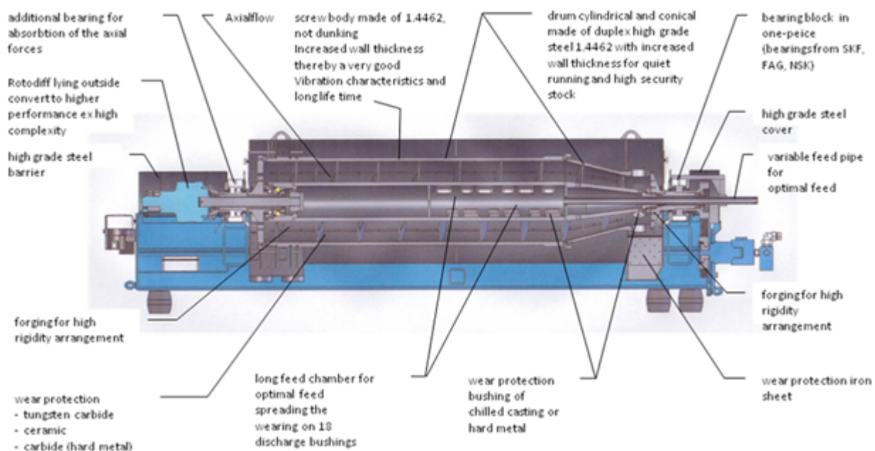
Рис 1. Устройство типичного трехфазного декантера компании Zentrifugen-Allianz
